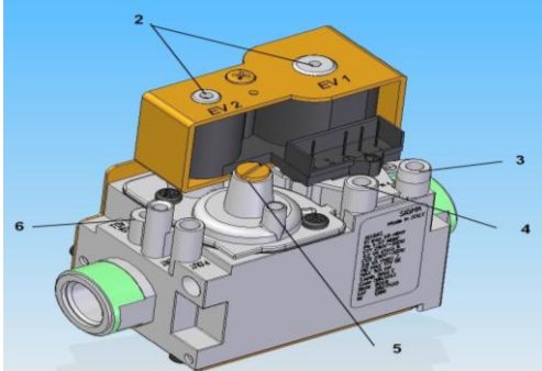
Εικόνα 4.2.1 Βαλβίδα Αερίου
