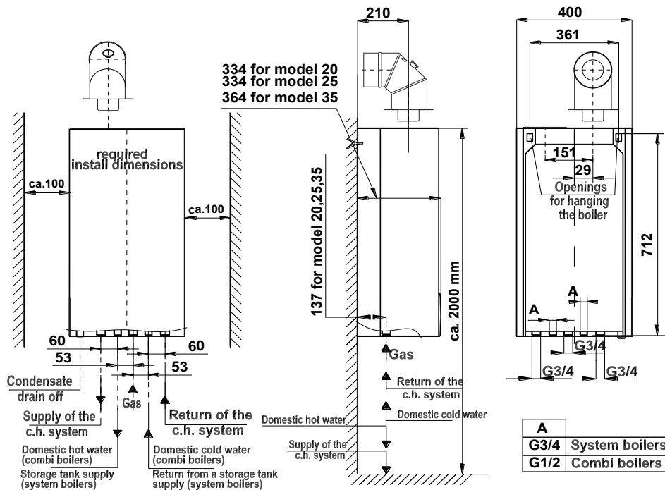
Εικόνα. 3.3.1 Διαστάσεις χρήσιμες για την Εγκατάσταση του ECOCONDENS Silver Plus
